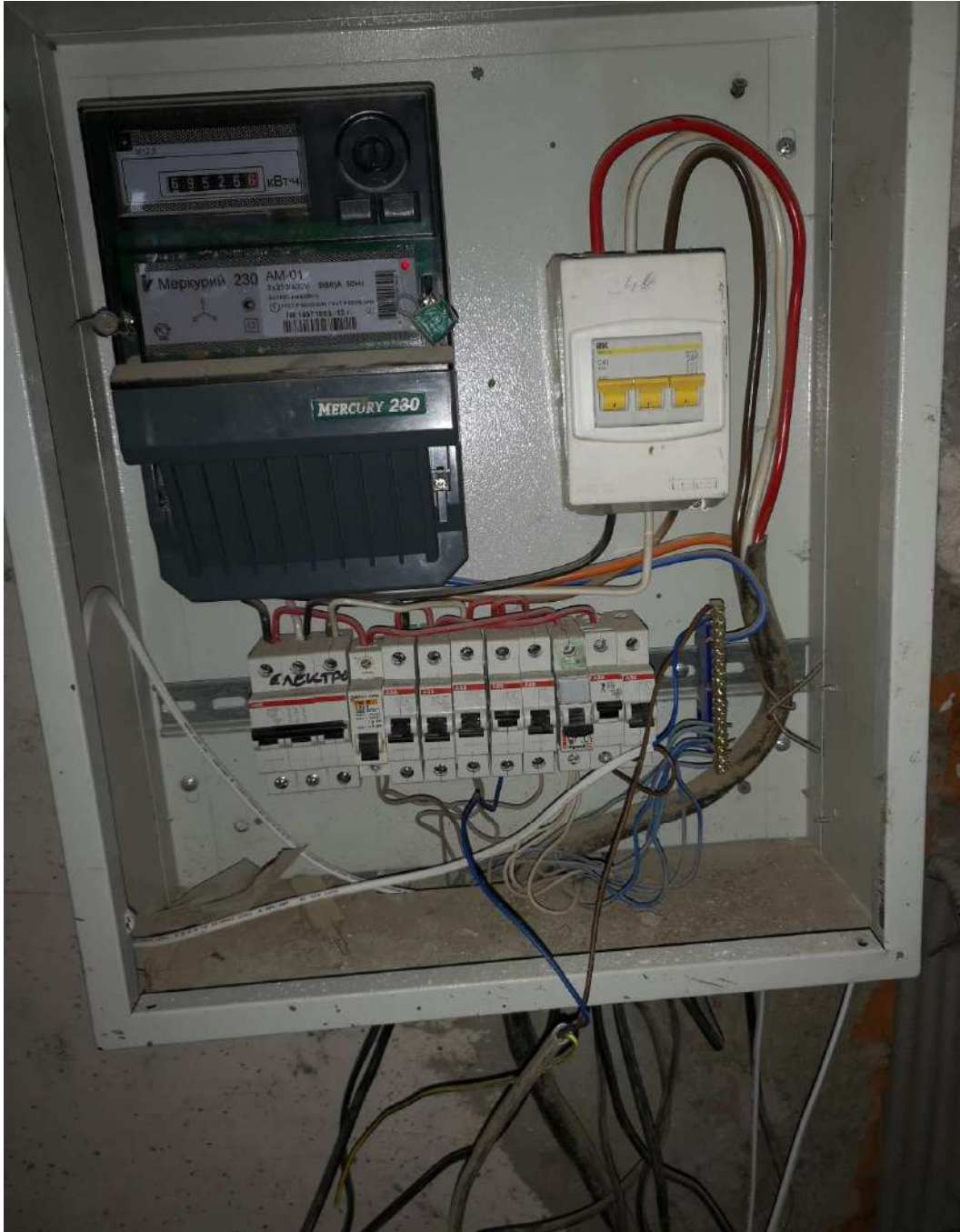
Электрический шкаф со счетчиком.
