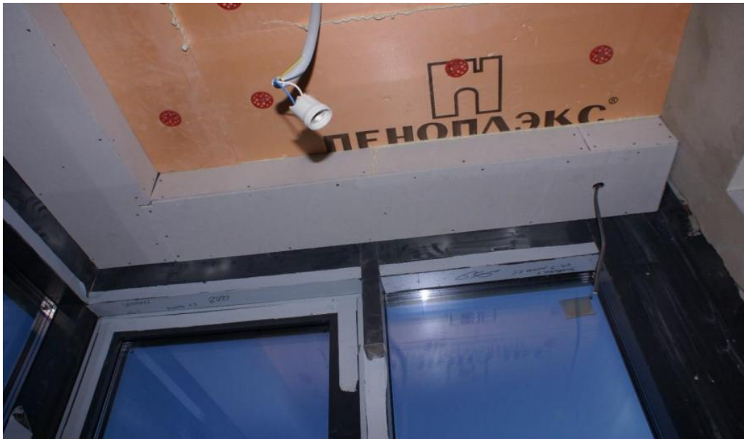
Устройство короба, 09.04.2018
