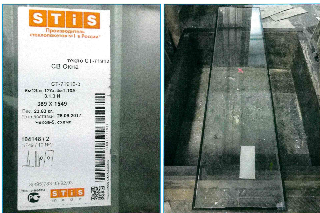
Рисунок 1. Этикетка стеклопакета и внешний вид образца после испытаний
